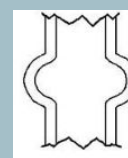
Panneaux avec nervures extérieures, entraxe 250mm
